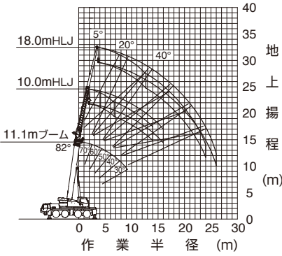
11.1mブーム+油圧チルトジブ
